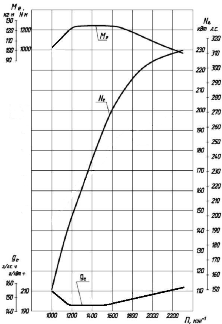
Рисунок 3у – Скоростная характеристика двигателя ЯМЗ-53613 на автобусах МАЗ
