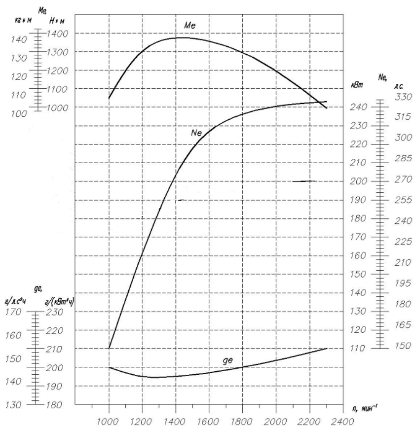
Рисунок 3н – Скоростная характеристика двигателя ЯМЗ-53676-10
