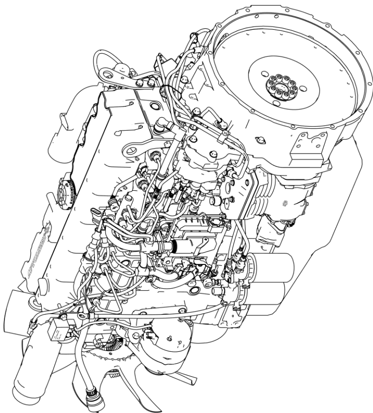
Рисунок 1л – Двигатель ЯМЗ-53642-20 – общий вид слева
