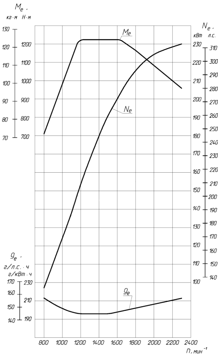
M_e – крутящий момент брутто; N_e – номинальная мощность брутто; g_e – удельный расход топлива; n – частота вращения коленчатого вала Рисунок 3е – Скоростная характеристика двигателя ЯМЗ-53601-40
