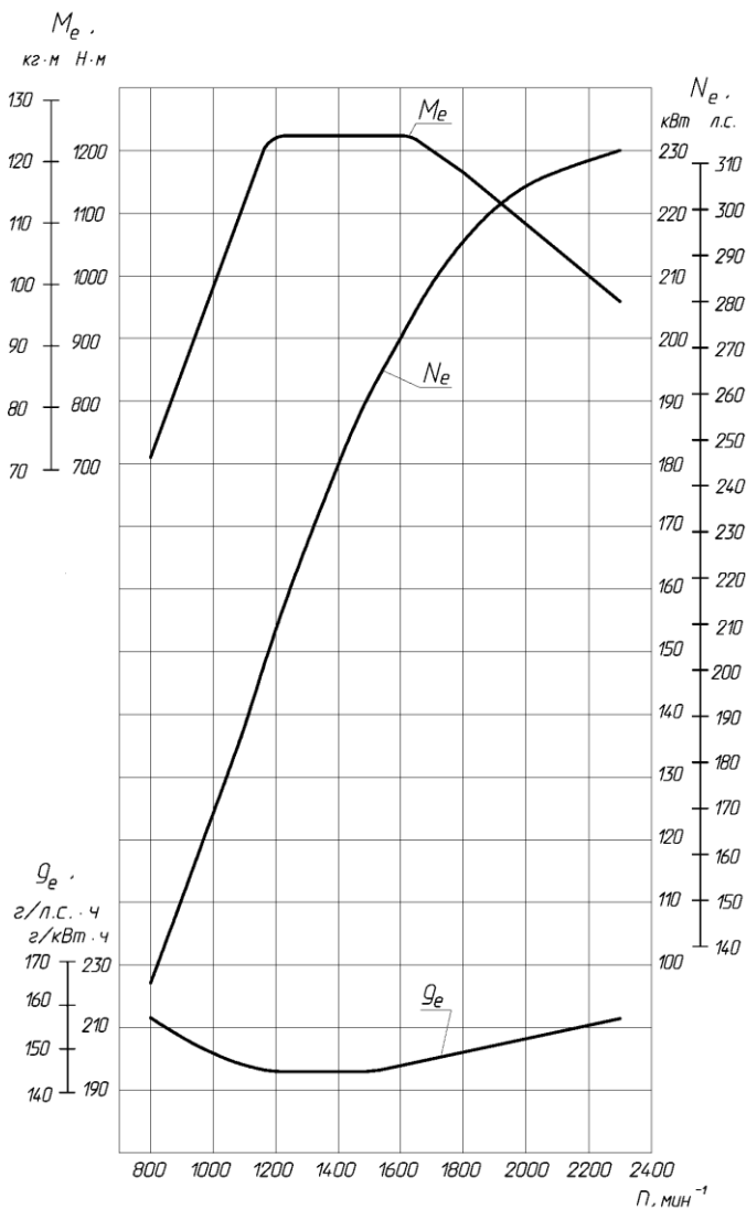
Рисунок 3г – Скоростная характеристика двигателя ЯМЗ-53613 на автобусах ЛиАЗ
