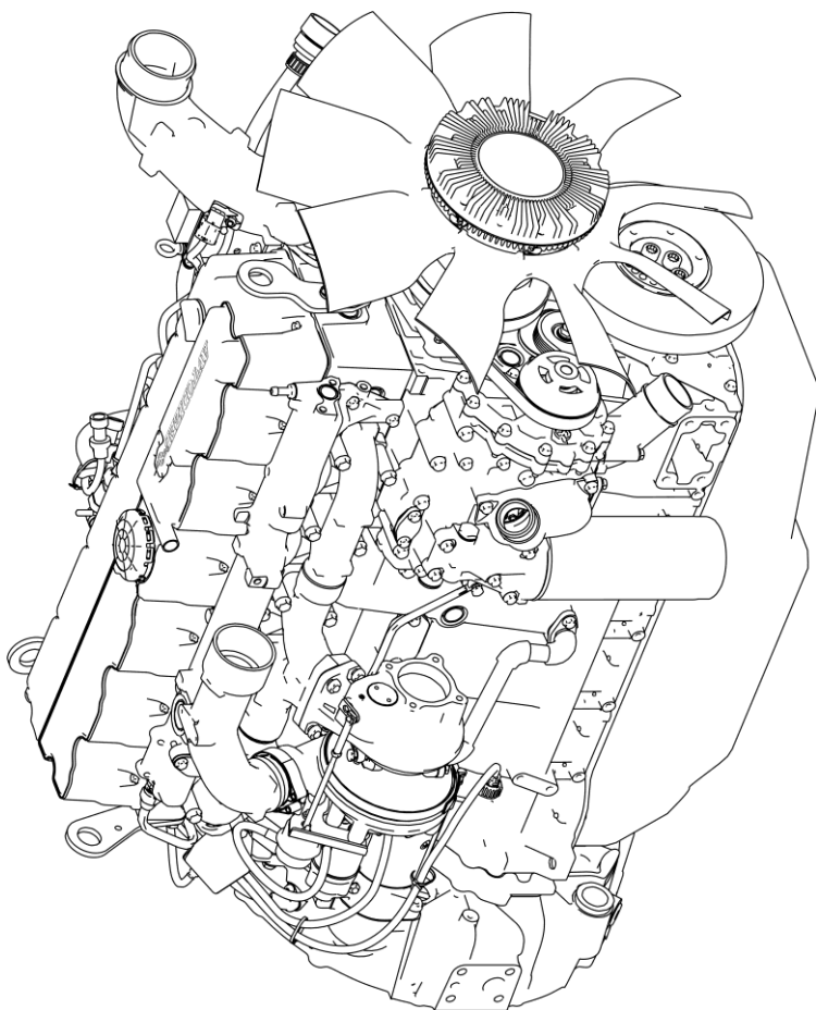
Рисунок. 1к – Двигатель ЯМЗ-53642-20 – общий вид справа
