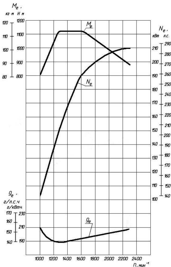
Рисунок 3г – Скоростная характеристика двигателей ЯМЗ-53642, ЯМЗ-53642-10
