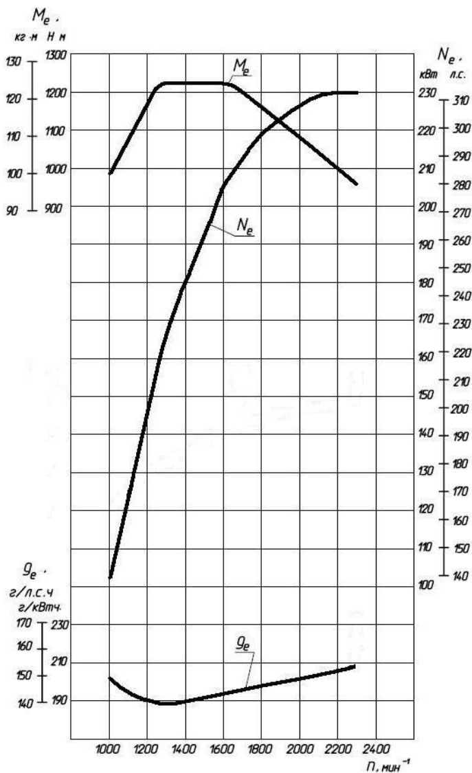
Рисунок 3б – Скоростная характеристика двигателей ЯМЗ-53602, ЯМЗ-53602-10
