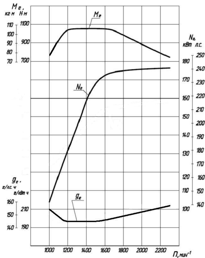
Рисунок 3з – Скоростная характеристика двигателей ЯМЗ-53631
