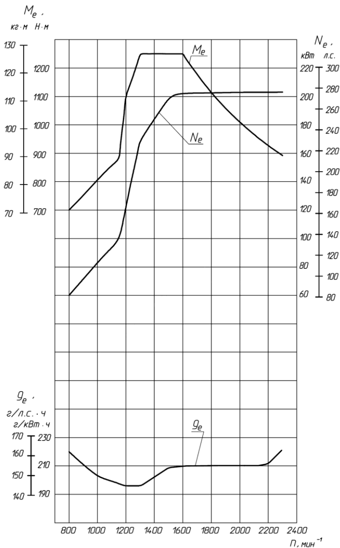
Рисунок 3к – Скоростная характеристика двигателя ЯМЗ-536111-40
