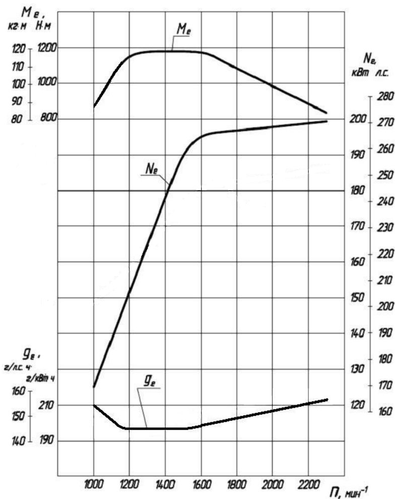
Рисунок 3ж – Скоростная характеристика двигателей ЯМЗ-53611
