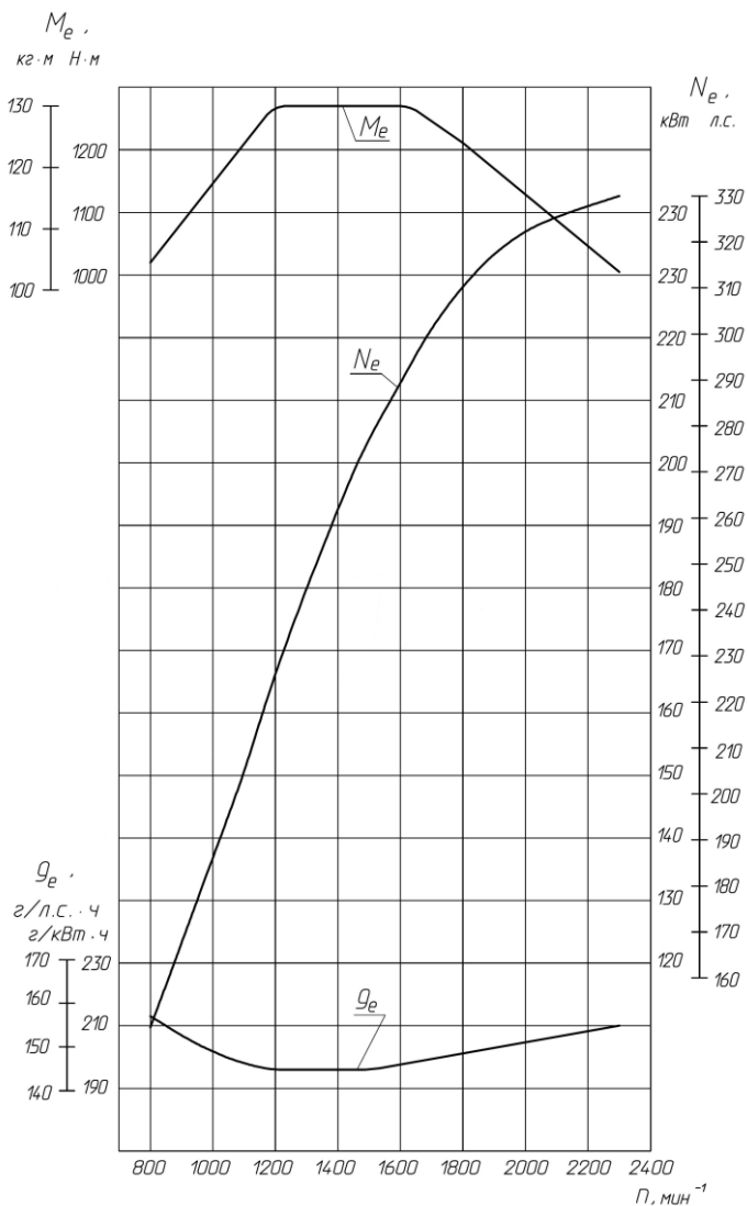
Рисунок 3м – Скоростная характеристика двигателей ЯМЗ-53603, ЯМЗ-53603-10
