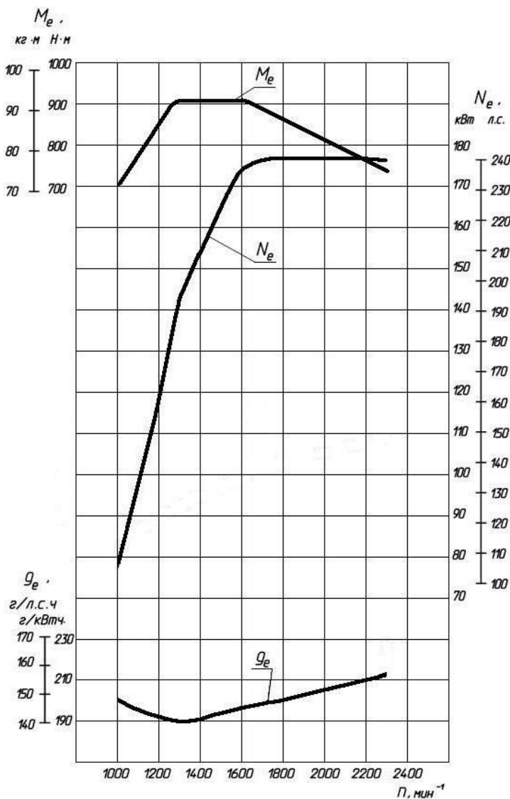
Рисунок 3в – Скоростная характеристика двигателей ЯМЗ-53622, ЯМЗ-53622-10
