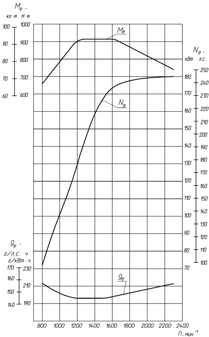
Рисунок 3л – Скоростная характеристика двигателя ЯМЗ-53621
