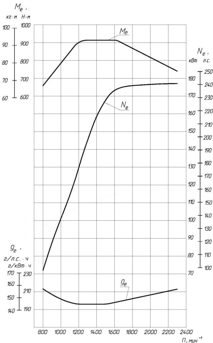
Рисунок 26 – Скоростная характеристика двигателя ЯМЗ-5362
