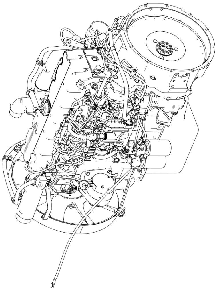
Рисунок 1 ж – Двигатель ЯМЗ-53602 – общий вид слева
