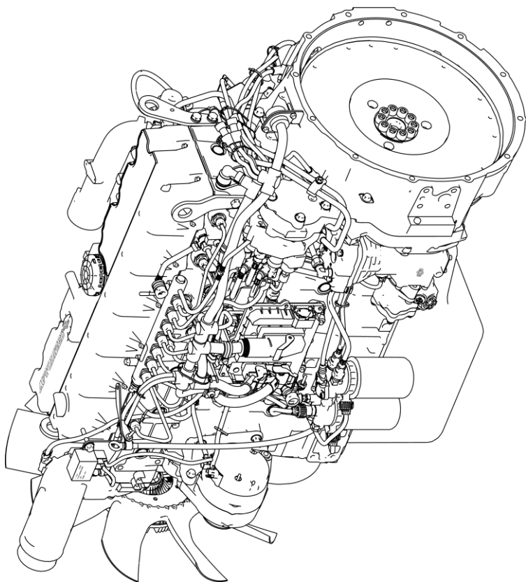
Рисунок 1и – Двигатель ЯМЗ-53602-10 – общий вид слева
