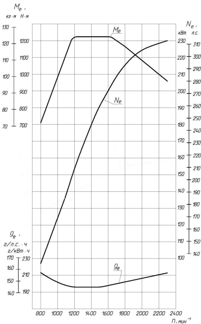
Рисунок 3а – Скоростная характеристика двигателя ЯМЗ-536-40
