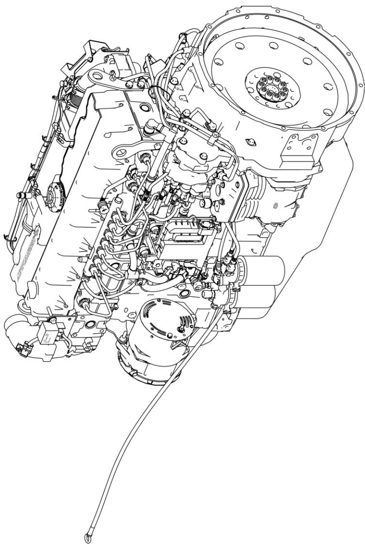
Рисунок 1д – Двигатель ЯМЗ-5362 – общий вид слева
