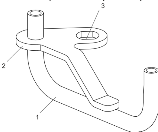
Рисунок 15 – Форсунка масляного охлаждения поршня
