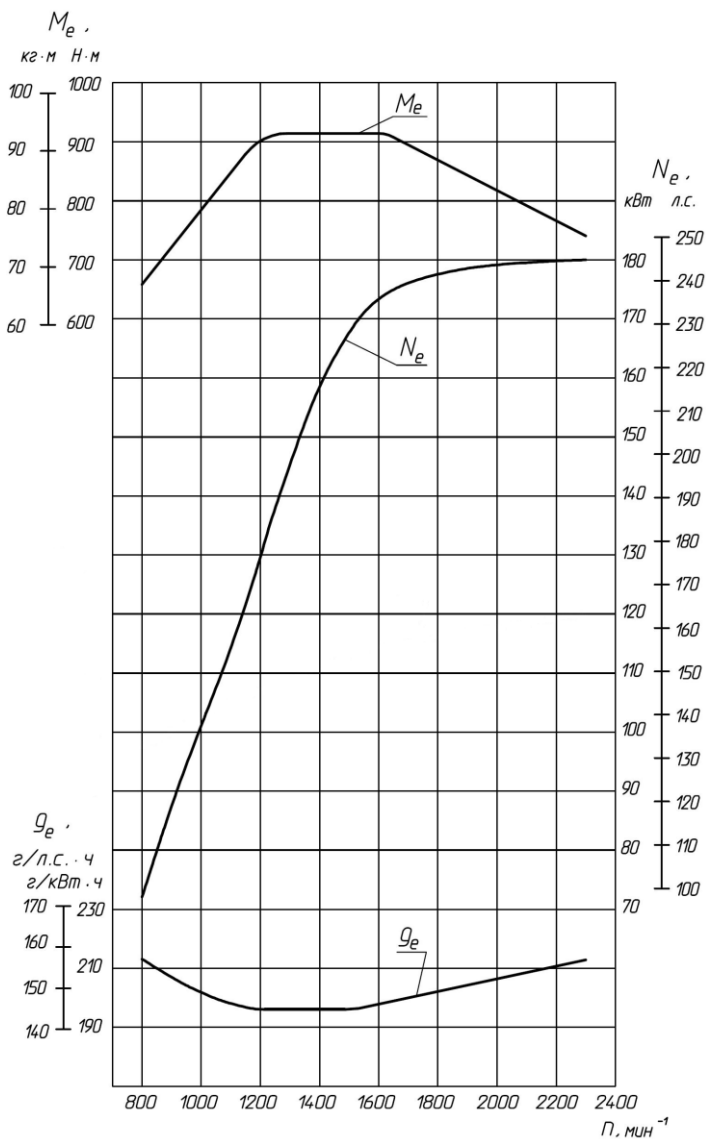
Рисунок 3х – Скоростная характеристика двигателей ЯМЗ-53663
