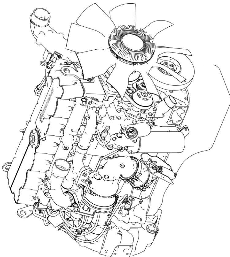
Рисунок 13 – Двигатель ЯМЗ-53602-10 – общий вид справа
